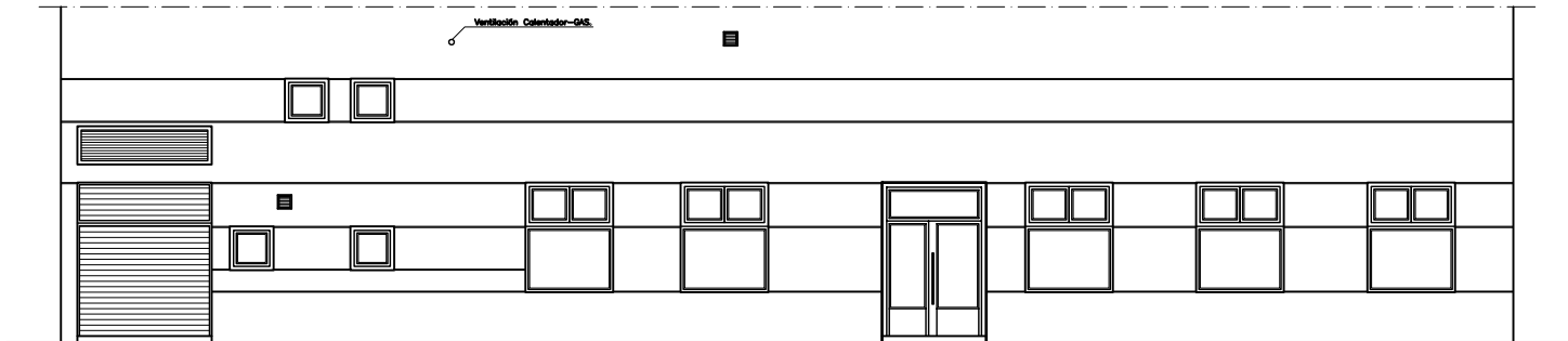
ALZADO PRINCIPAL.
