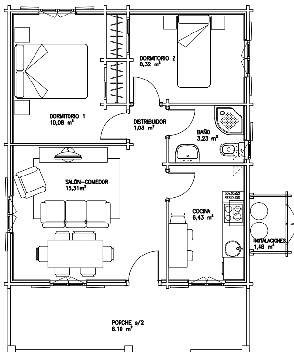
PLANTA BAJA.
