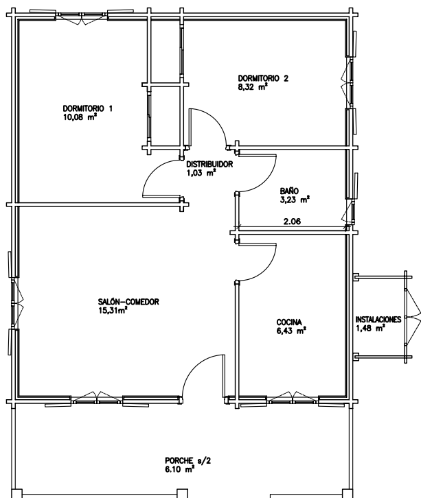
PLANTA BAJA.
